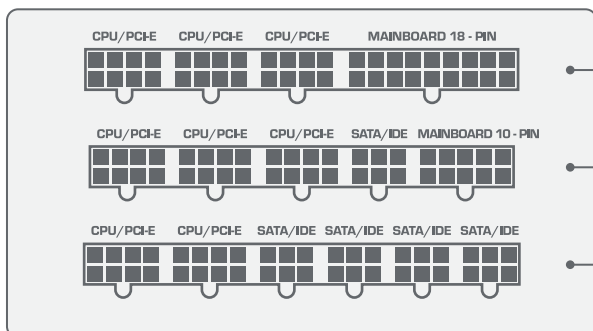
Supremo FM2 Gold 750W
