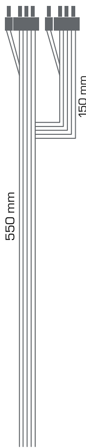
PCI-E (6+2 - PIN) VGA
